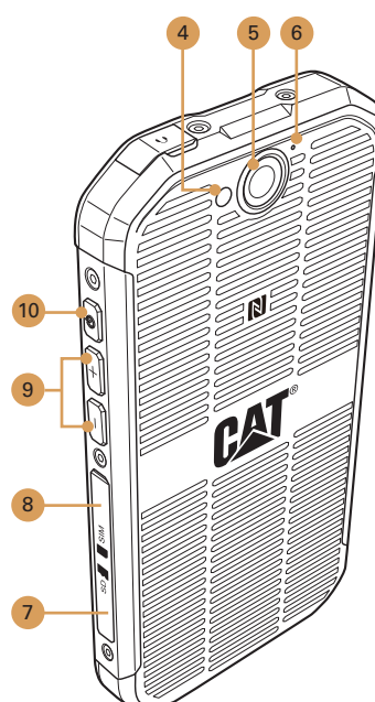
SEDD BAKIFRÅN
