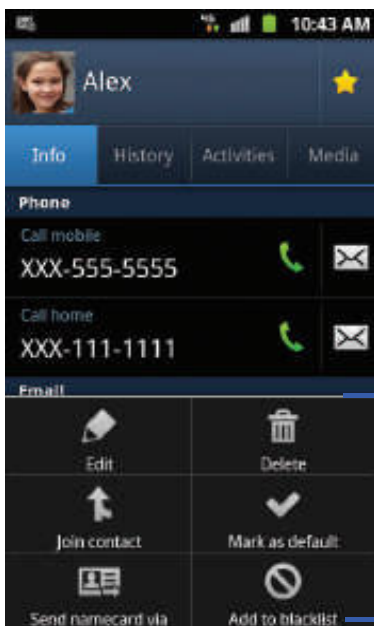
Sub-Menu items
